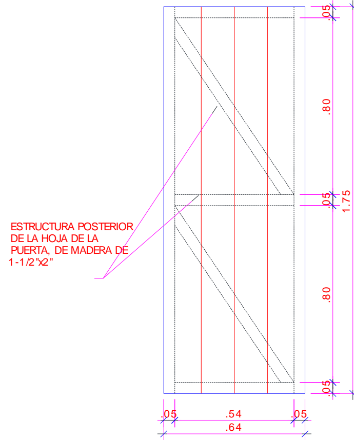
VISTA_POSTERIOR_DE_LA_PUERTA
